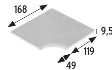
8 Esq. int. canto romo Bullnose int. corner
