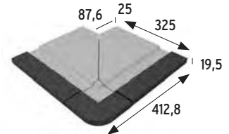
B33 SPORT edge ext. corner
