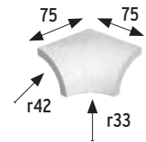
4 Esq. int. rinconera Internal mitre
