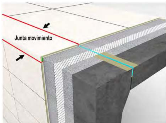
プール縁部とプール内側躯体の間に設けられた可動目地 (赤色表示)
