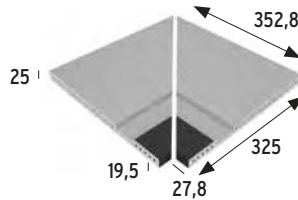
B33 SPORT edge int. corner
