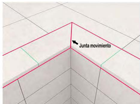
プールのコーナー部に設けられた可動目地 (赤色表示)
