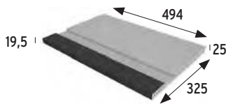
B33 SPORT edge
