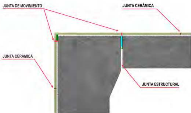
COLOCACIÓN BORDE ENRASADO AL REVESTIMIENTO. LAYING EDGE FLUSH WITH THE CLADDING.
