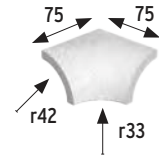
5 Esq. int. rinconera Internal mitre
