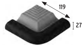
Finnish edge external corner
