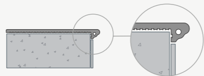
階段フィオレンティーノ踏面 Stairs fiorentino tread.
